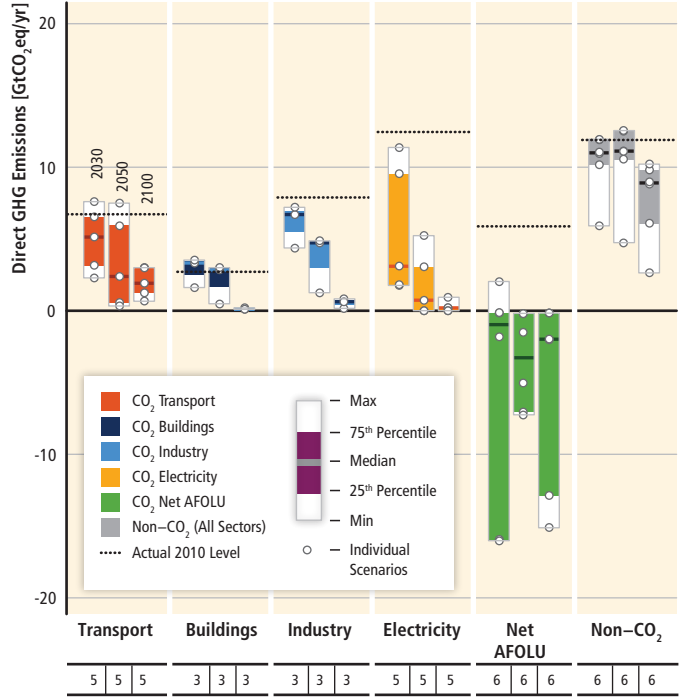
450 ppm CO 2 eq without CCS
